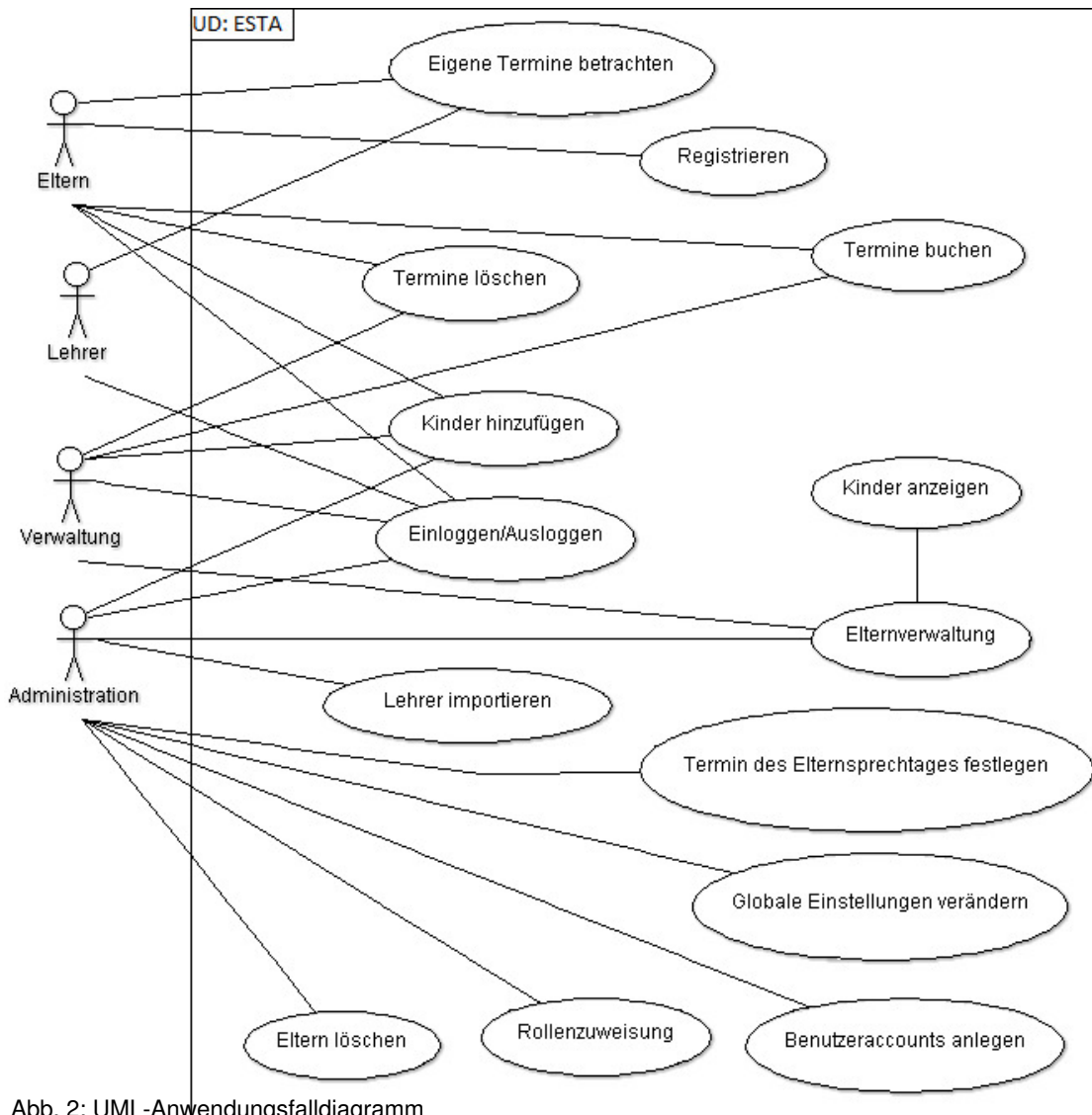
Abb. 2: UML-Anwendungsfalldiagramm
