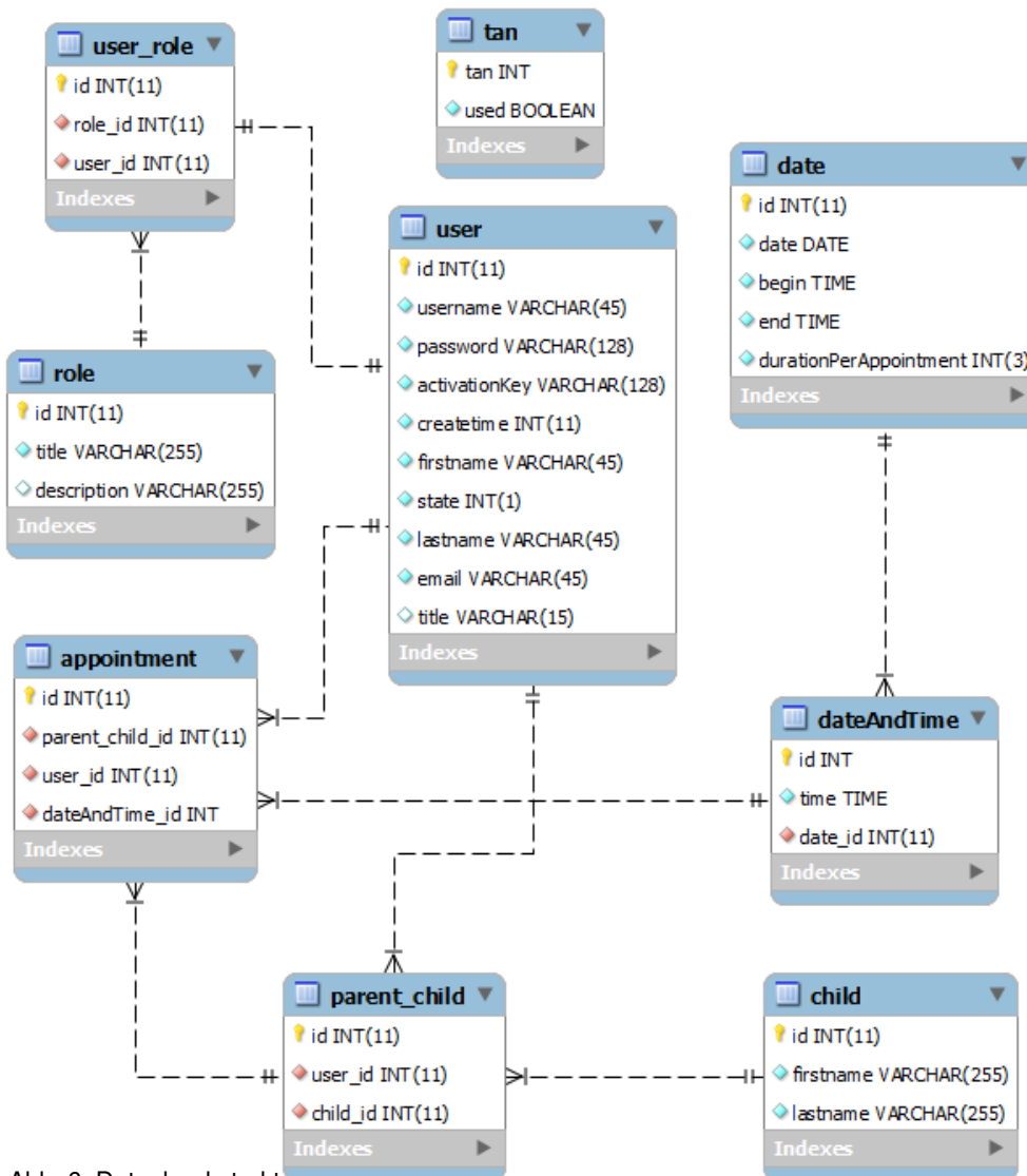
Abb. 6: Datenbankstruktur
