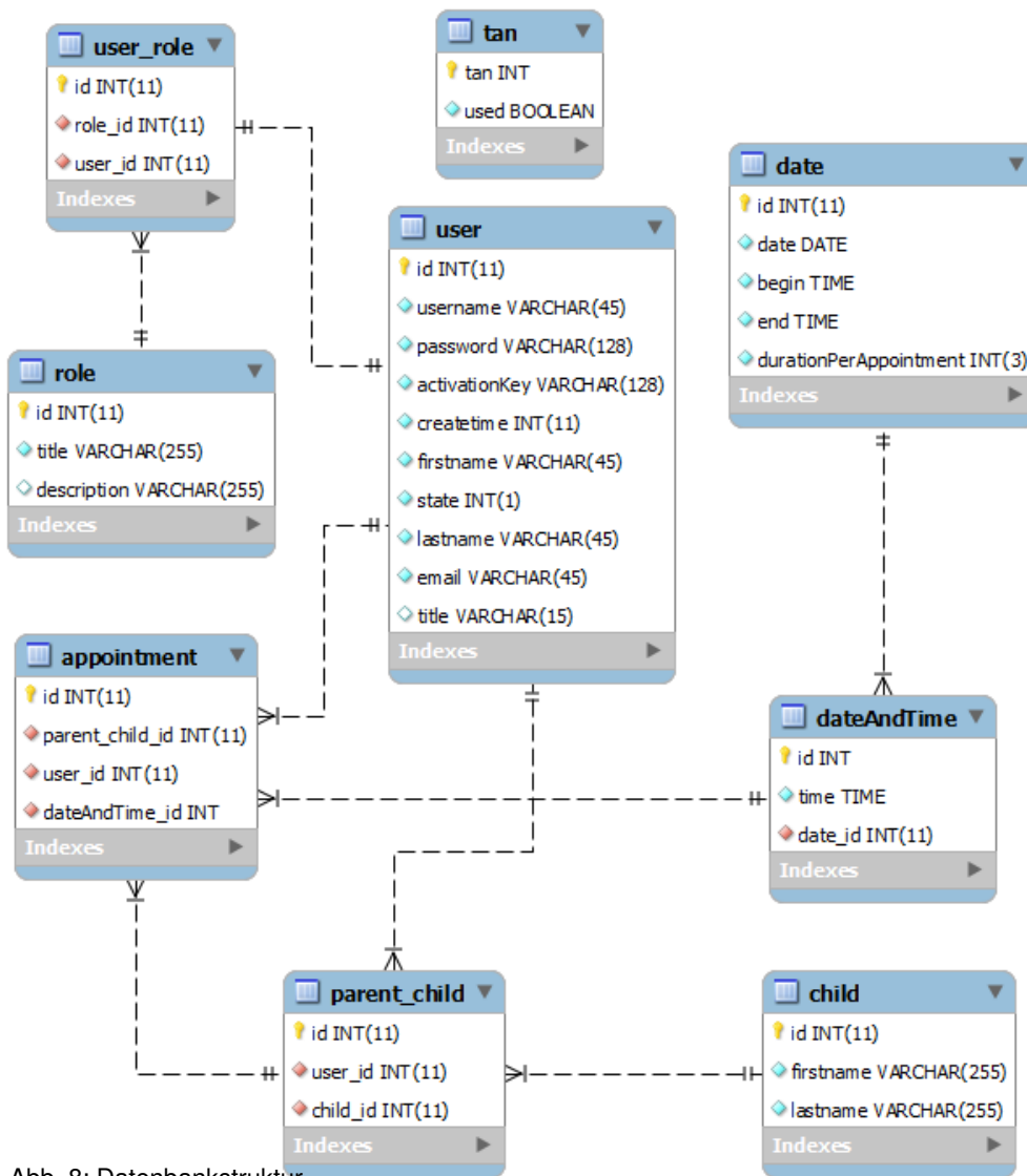
Abb. 8: Datenbankstruktur
