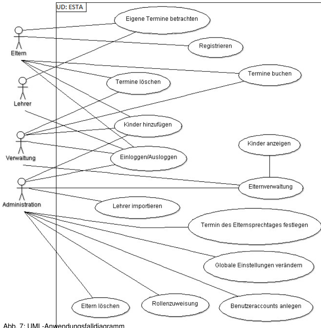
Abb. 7: UML-Anwendungsfalldiagramm
